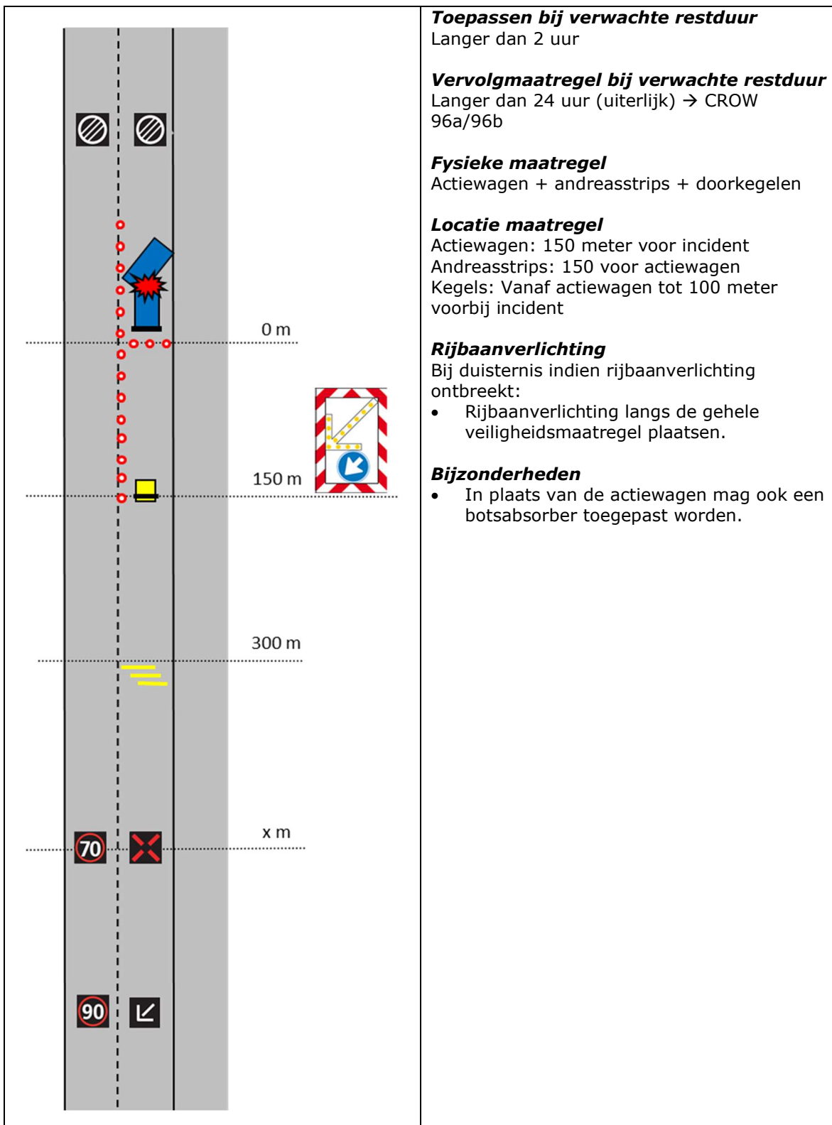
Figuur 3.2 Veiligheidsmaatregel fase 2 op auto(snel)wegen met verkeerssignalering
