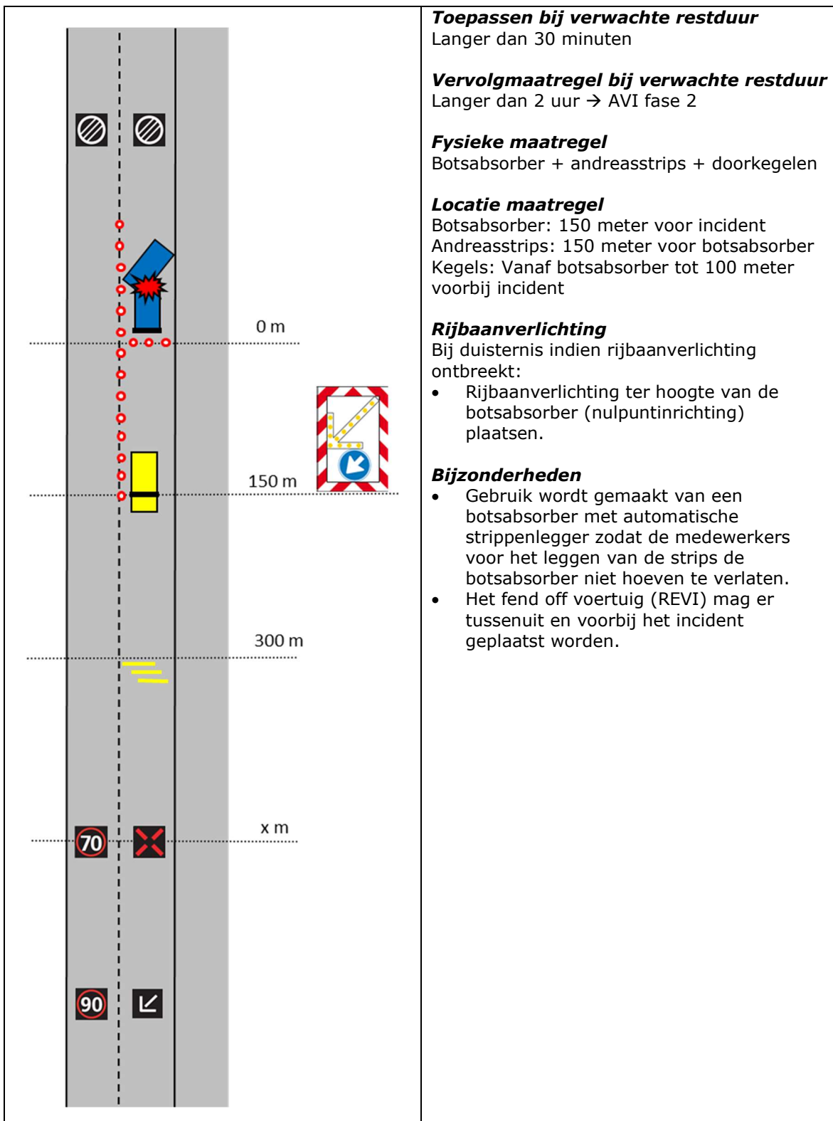
Figuur 3.1 Veiligheidsmaatregel fase 1 op auto(snel)wegen met verkeerssignalering
