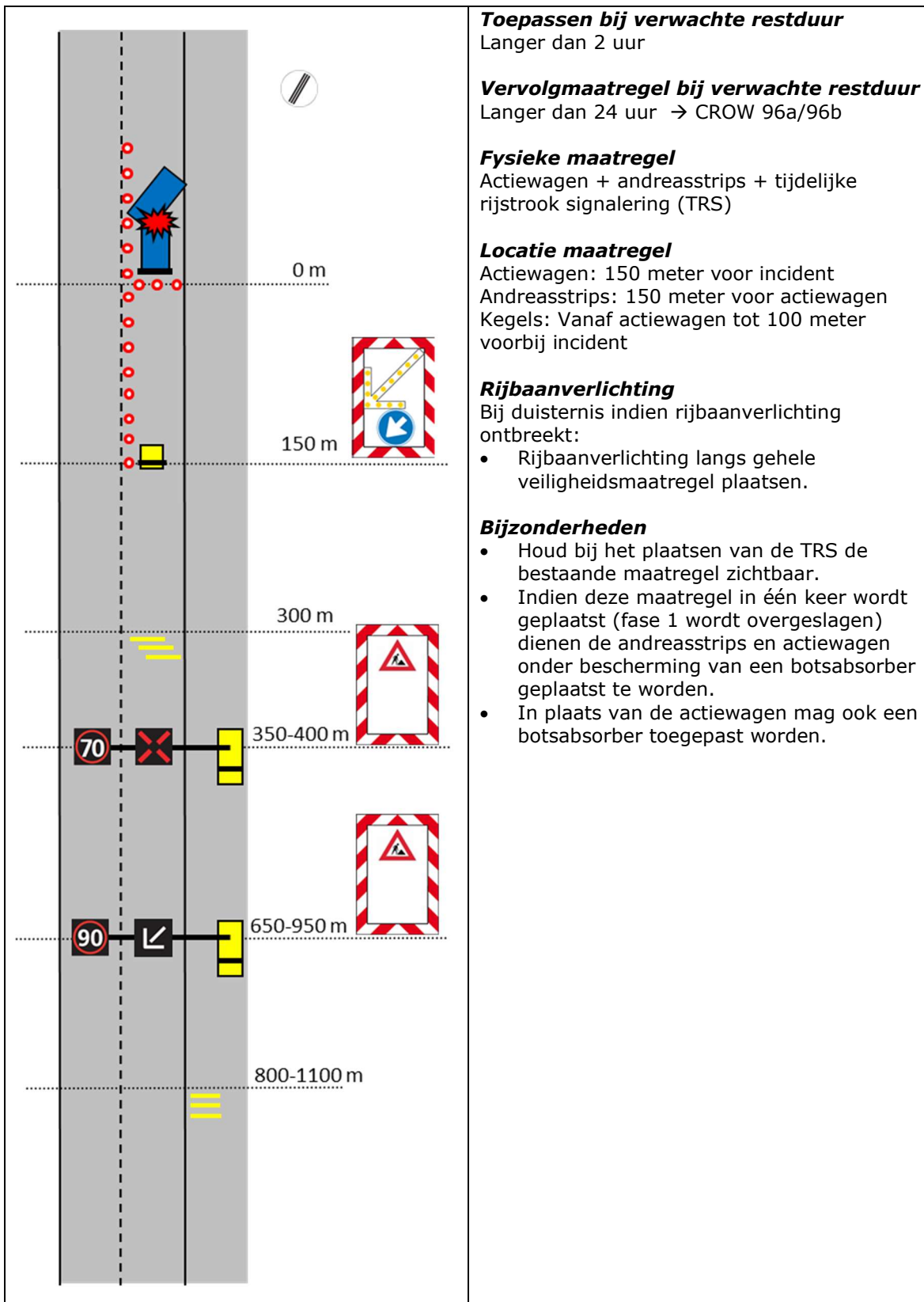
Figuur 4.2 Veiligheidsmaatregel fase 2 op auto(snel)wegen zonder verkeerssignaling
